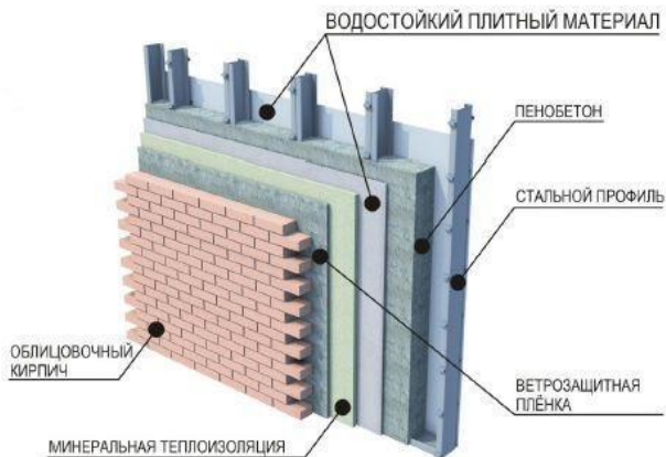
Рисунок 5. Стеновая панель с пенобетоном [30]
