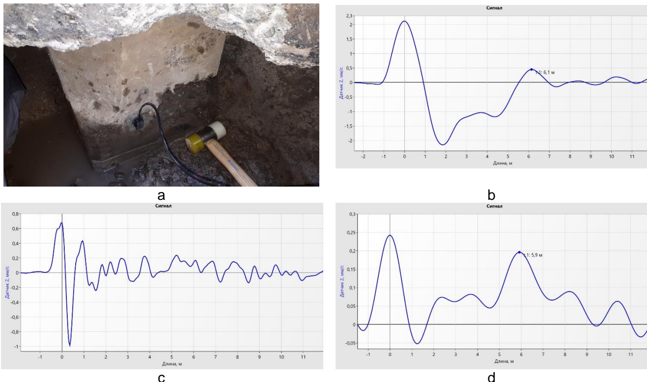
Рисунок 9 - Ленточный ростверк жилого здания. Забивные сваи длиной 6 м: а - боковой датчик, установленный на сваю, удар наносится по штрабе; б - сигнал, полученный при низкочастотном воздействии; с - сигнал, полученный при высокочастотном воздействии; д - высокочастотный сигнал после фильтрации 1,2 кГц
