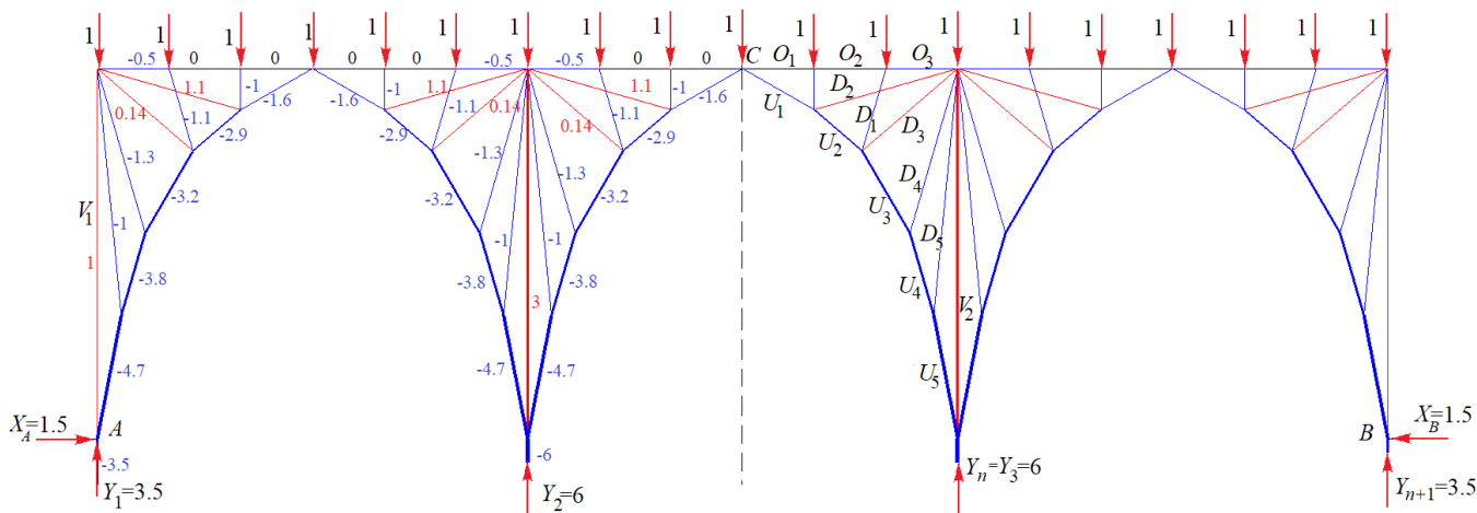
Рис. 4 – Распределение усилий в стержнях фермы, n = 3, a = h = 1\text{ м}
