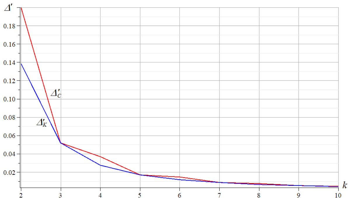
Рис. 5 – Зависимость прогибов в узлах С и К при равномерном нагружении от числа пролетов Fig. 5 – Dependence of deflections in nodes С and К under uniform loading on the number of spans
